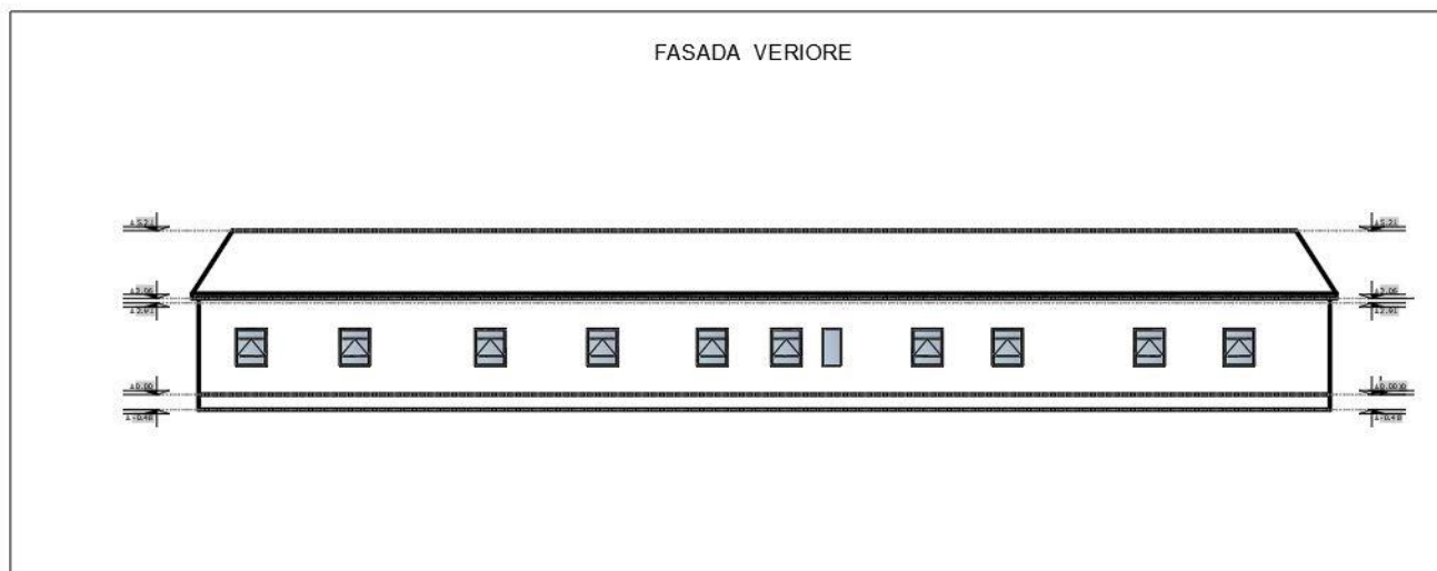
Figura 16. Fasada nga Veriu
