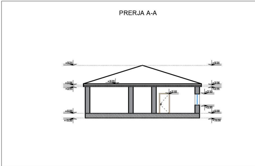
Figura 13. Prerja A-A
