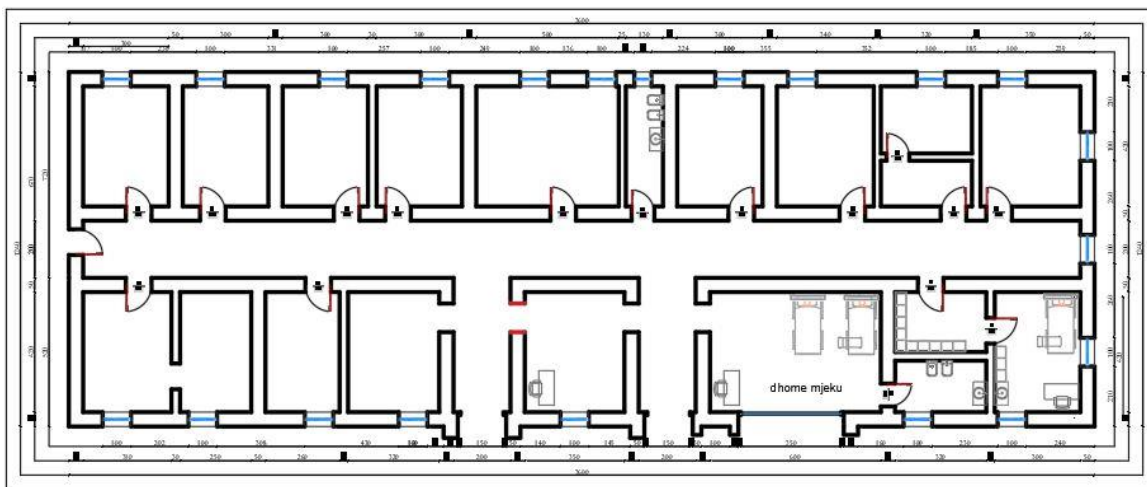
Figura 6. Planimetria e gjendjes ekzistuese
