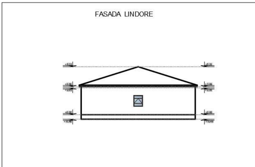
Figura 17. Fasada nga Lindja.
