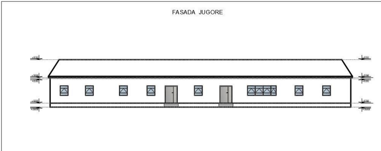
Figura 15. Fasada nga Jugu
