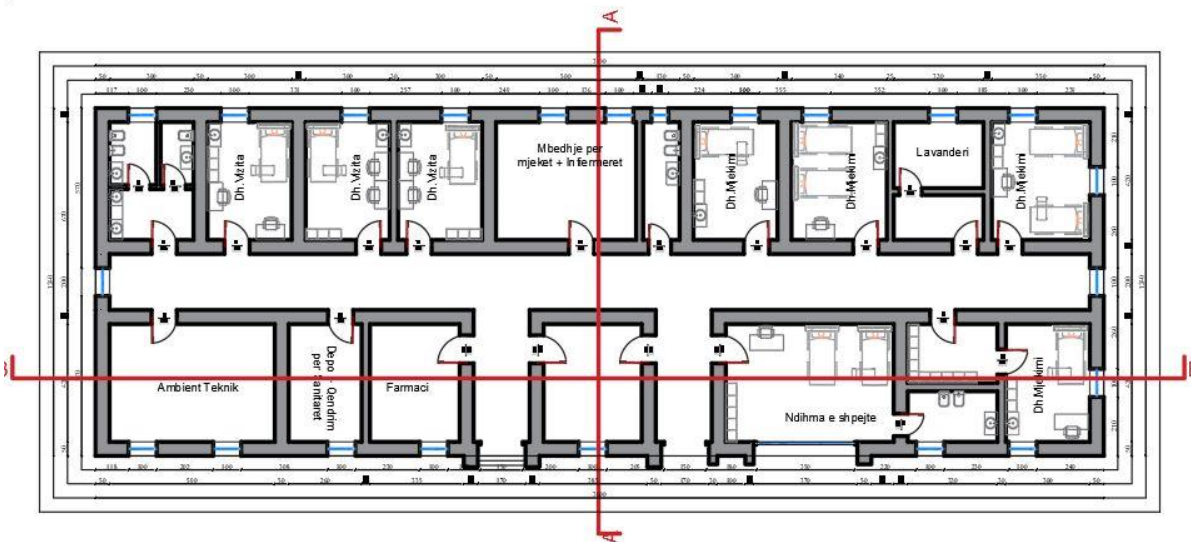
Figura 11. Planimetria e propozuar
