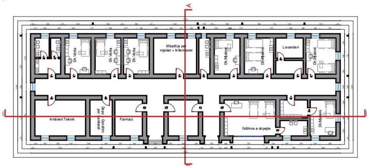
Figura 7. Planimetria e propozuar
